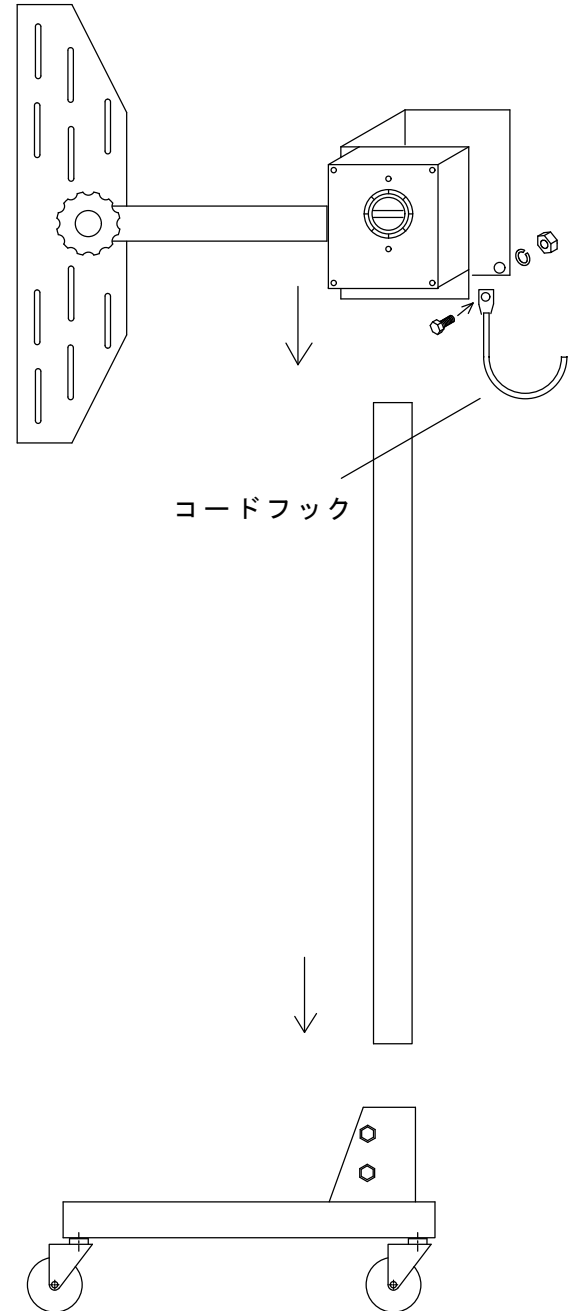
本体組立図
