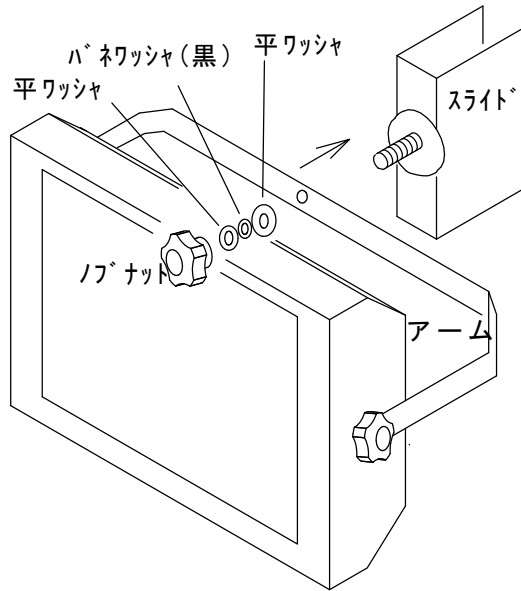
本体取付図
