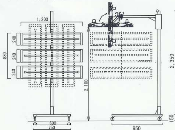
ポデー寸法図 (単位:mm)
